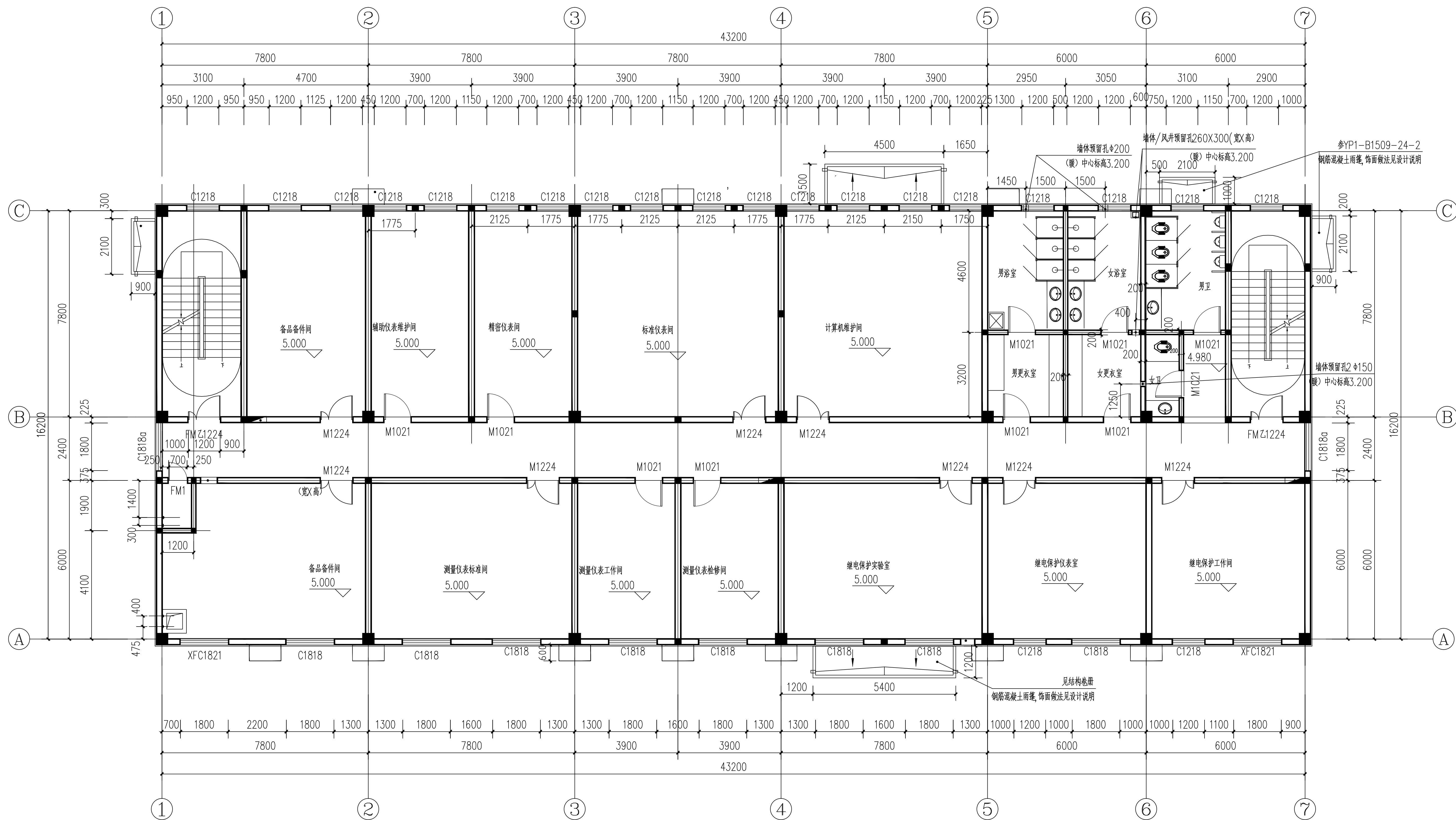
检修维护楼5.000m层平面布置图 1:100
