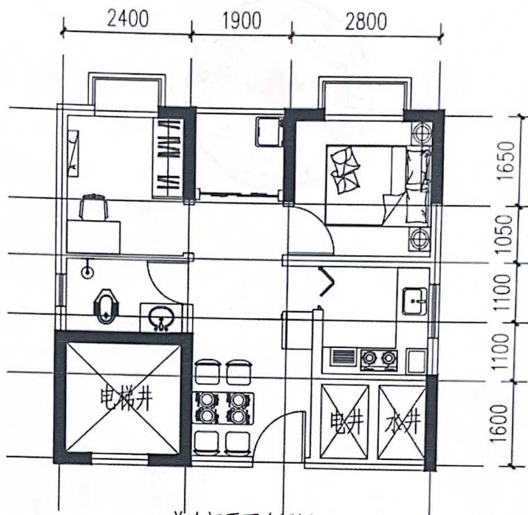
单人间平面布置图 1:100
